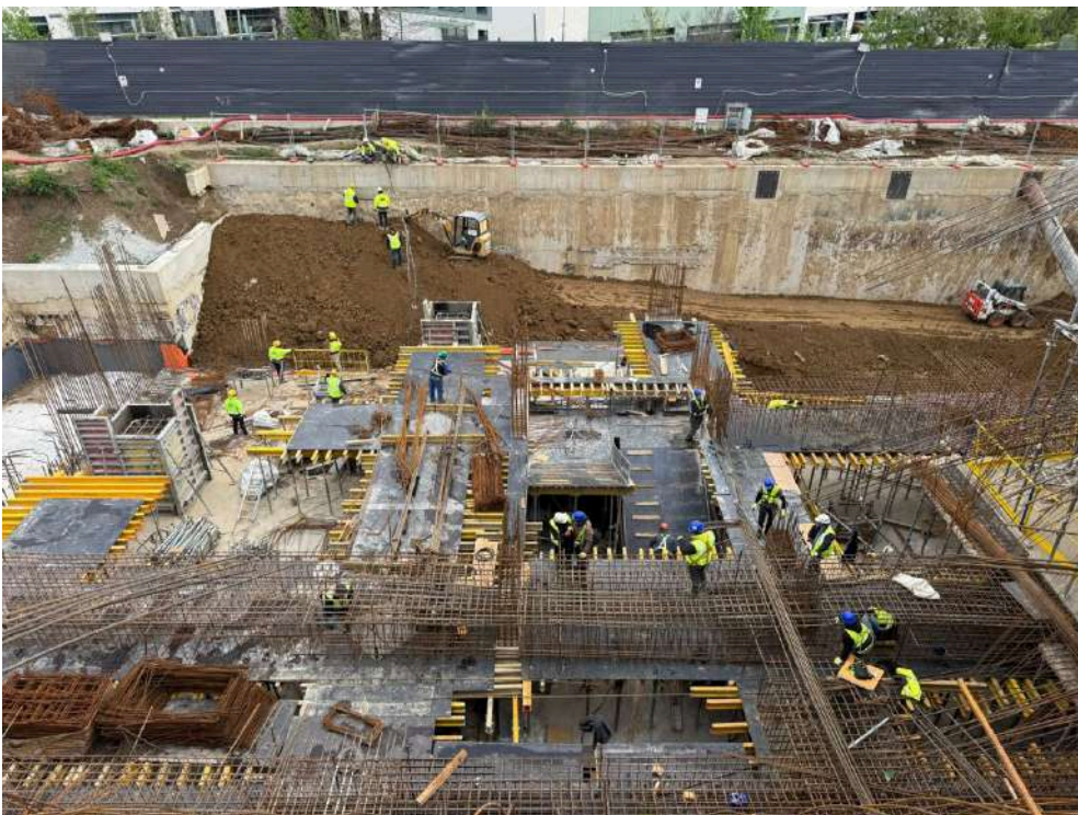
2026.04.22 - Vedere generala, zona MH
