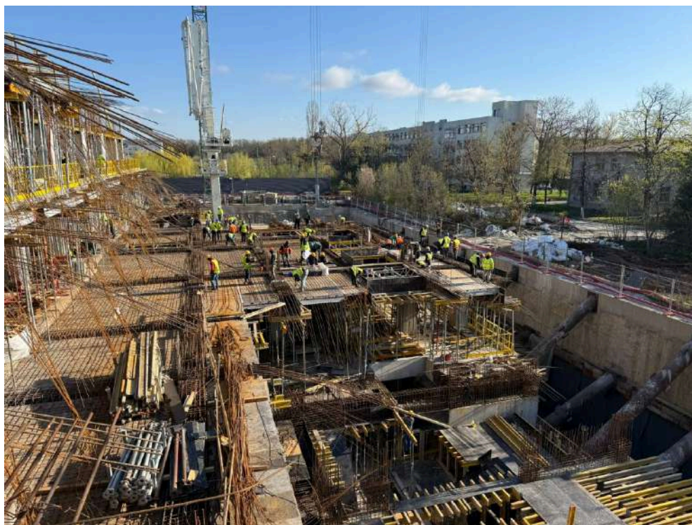
2026.04.08 - Vedere generala, zona MH
