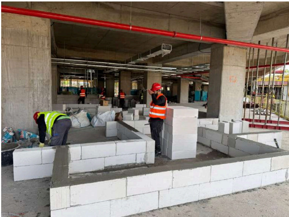
2026.04.21 - Executie pereti despartitori din BCA
