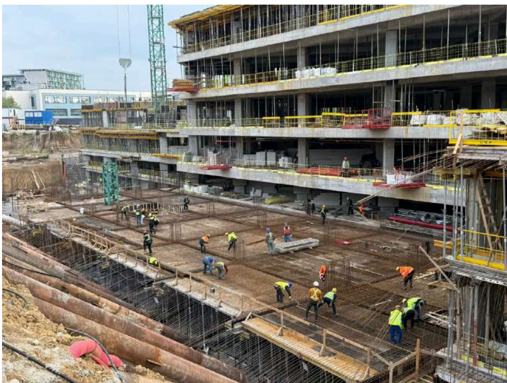
2026.04.22 - Lucrari de cofrare, armare, zona MH
