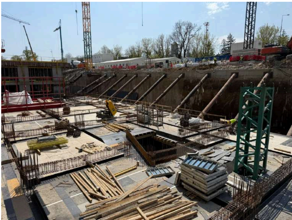
2026.04.17 - Lucrari de cofrare, armare, zona MH
