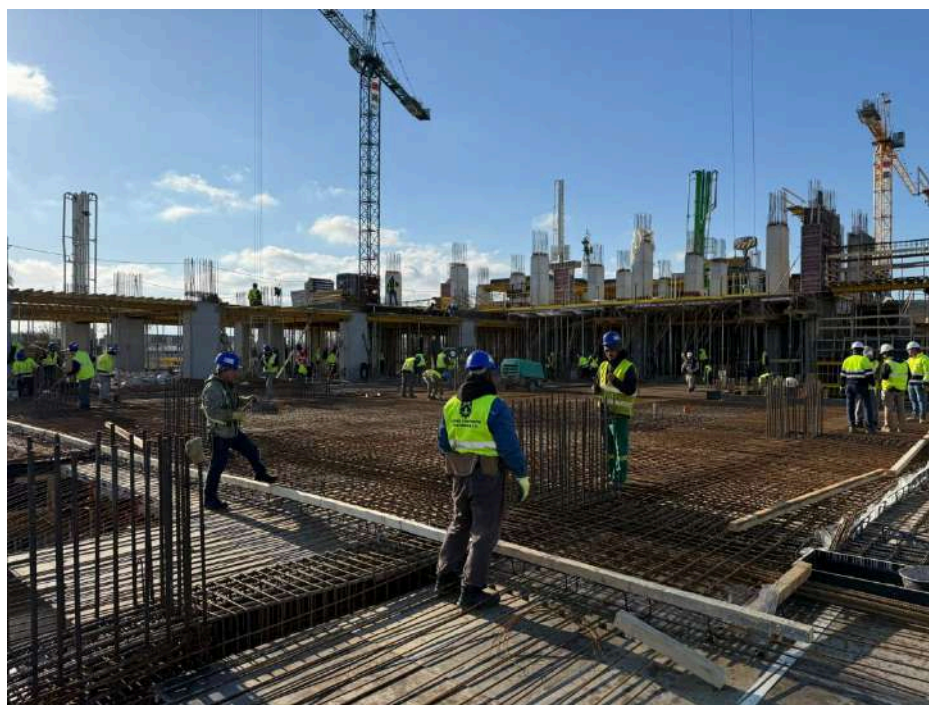
2026.04.08 - Lucrari de cofrare, armare, zona MH
