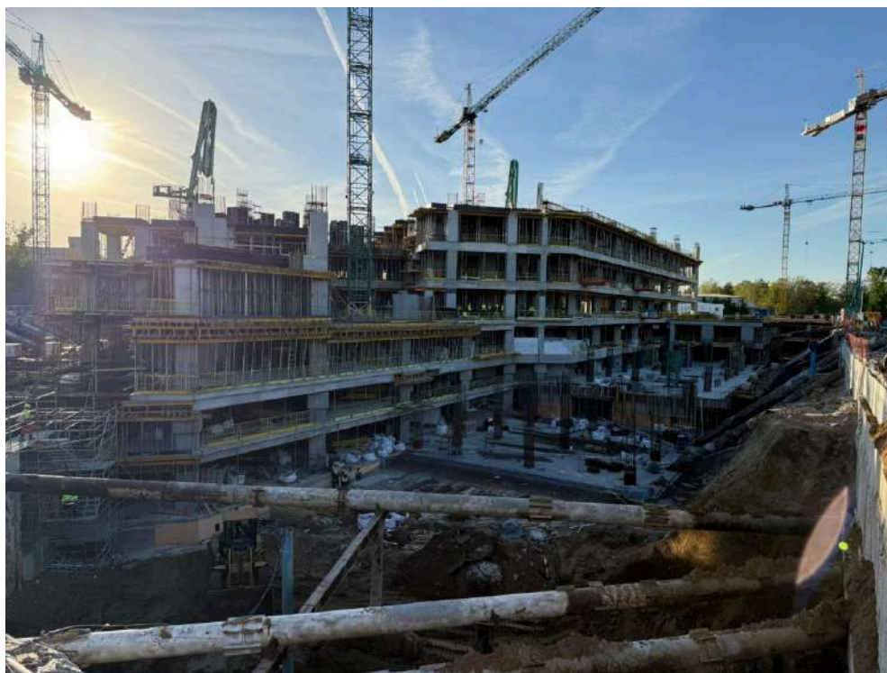
2026.04.27 - Vedere generala, zona MH
