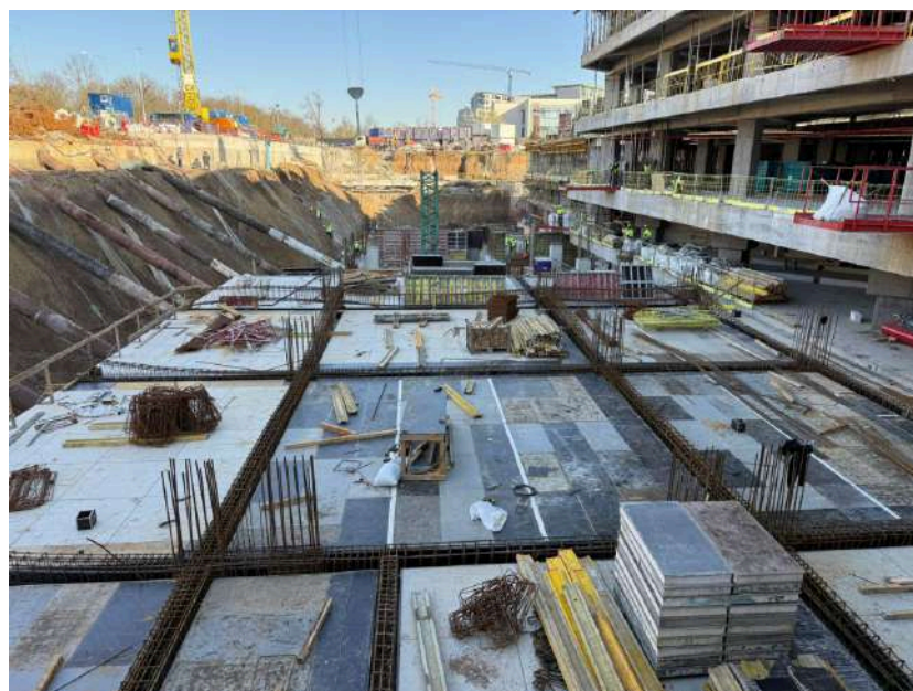
2026.04.09 - Lucrari de cofrare, armare, zona MH
