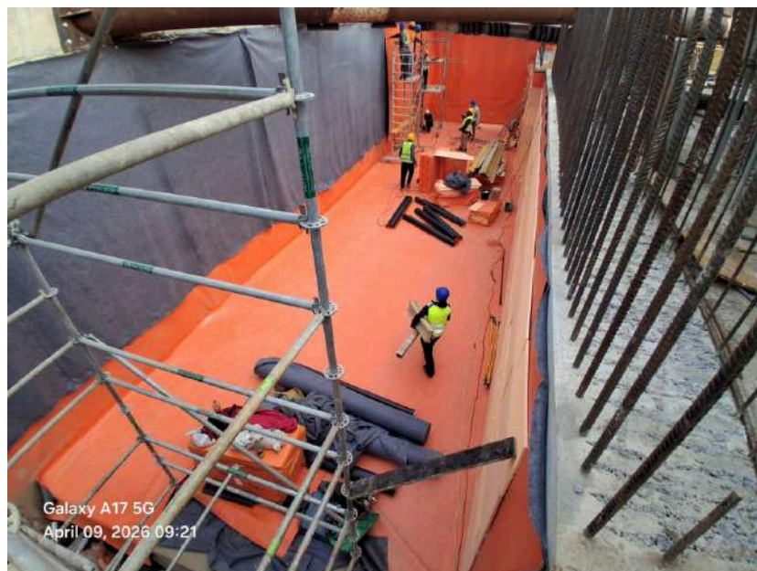
2026.04.09 - Sistem complet de izolație incintă
