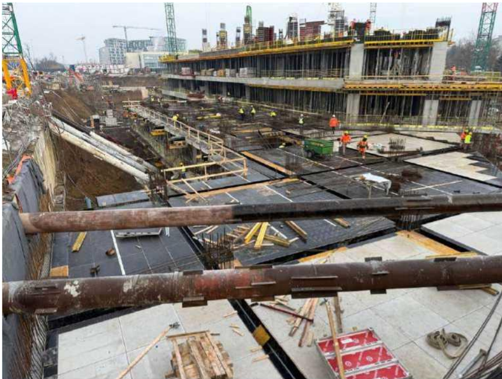
2026.03.01 - Lucrari de cofrare, armare, zona MH
